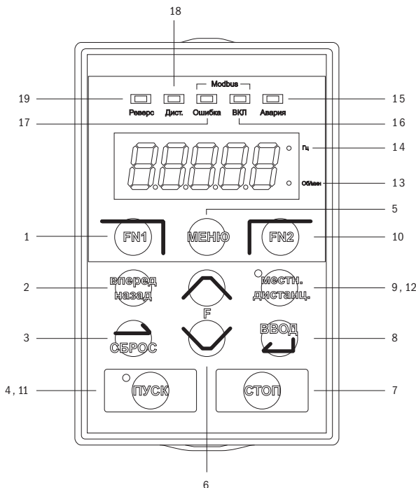
Рисунок 5.1.1. Кнопочная панель
